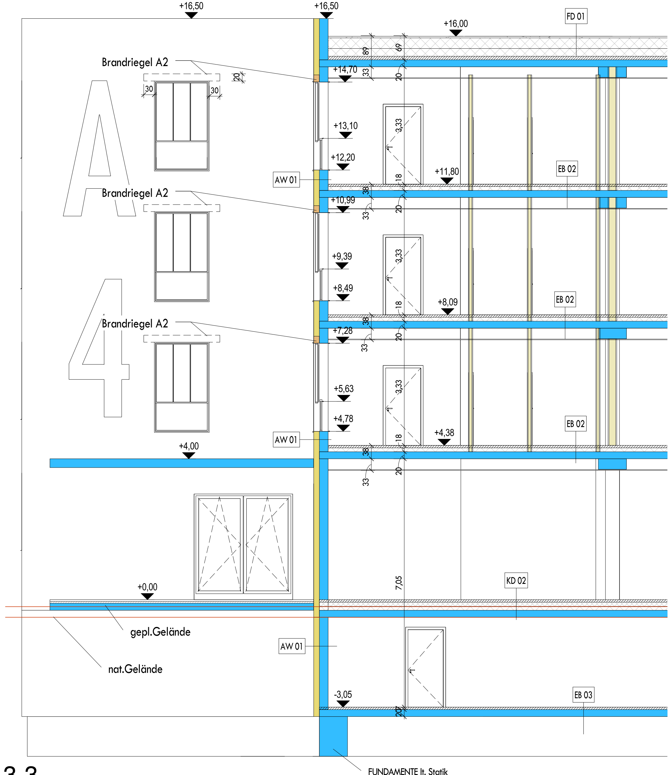
3-3 M 1 : 100
