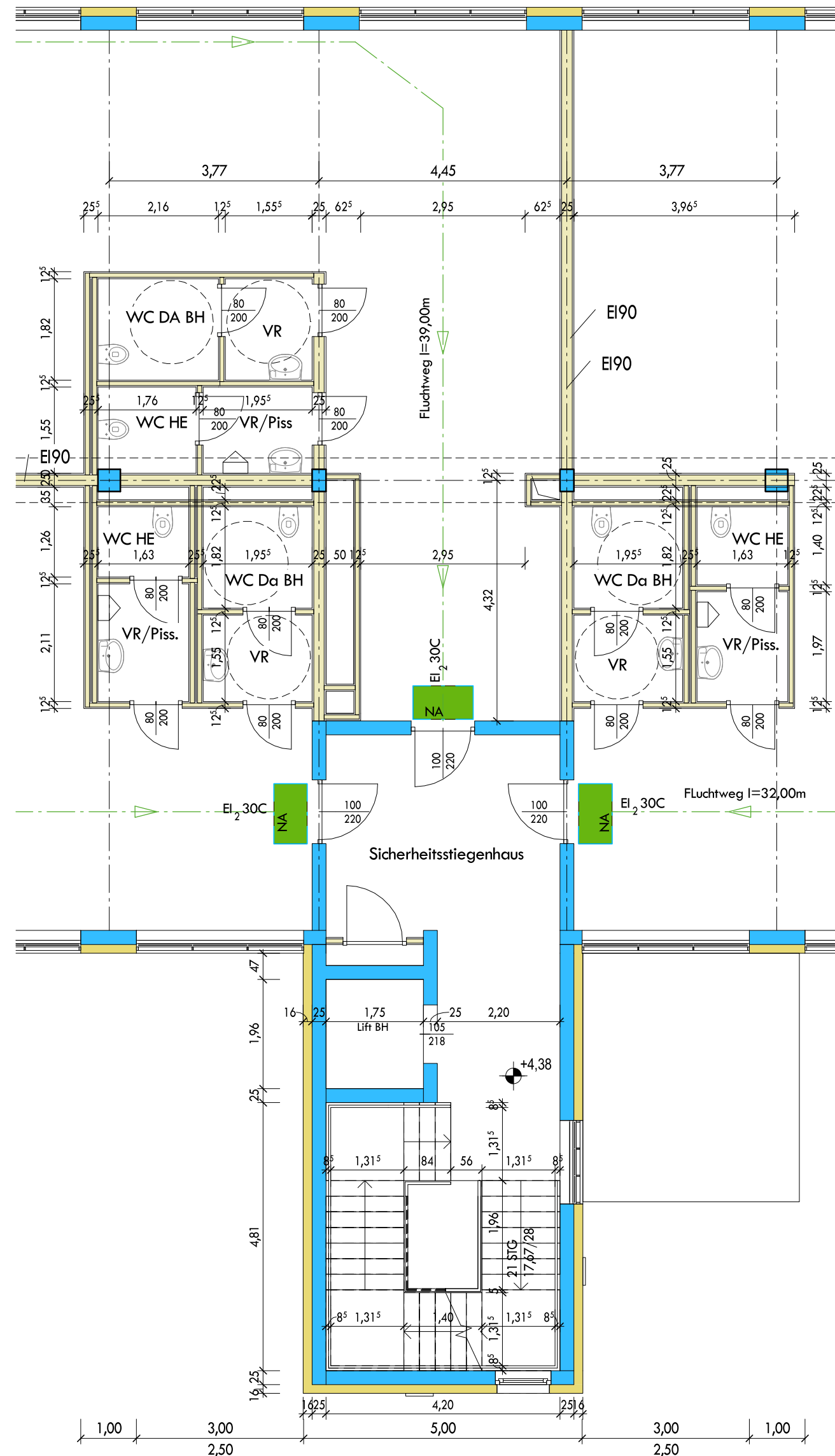
BT_A4_1-3 OG Sanitärgruppe Stiegenhaus
