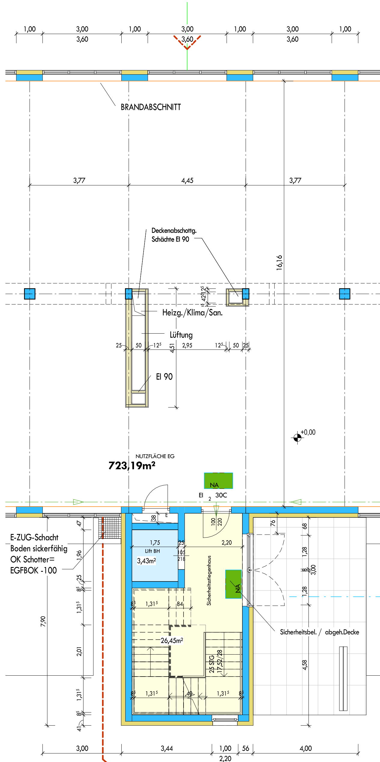
BT_A4_EG Sanitärgruppe Stiegenhaus
