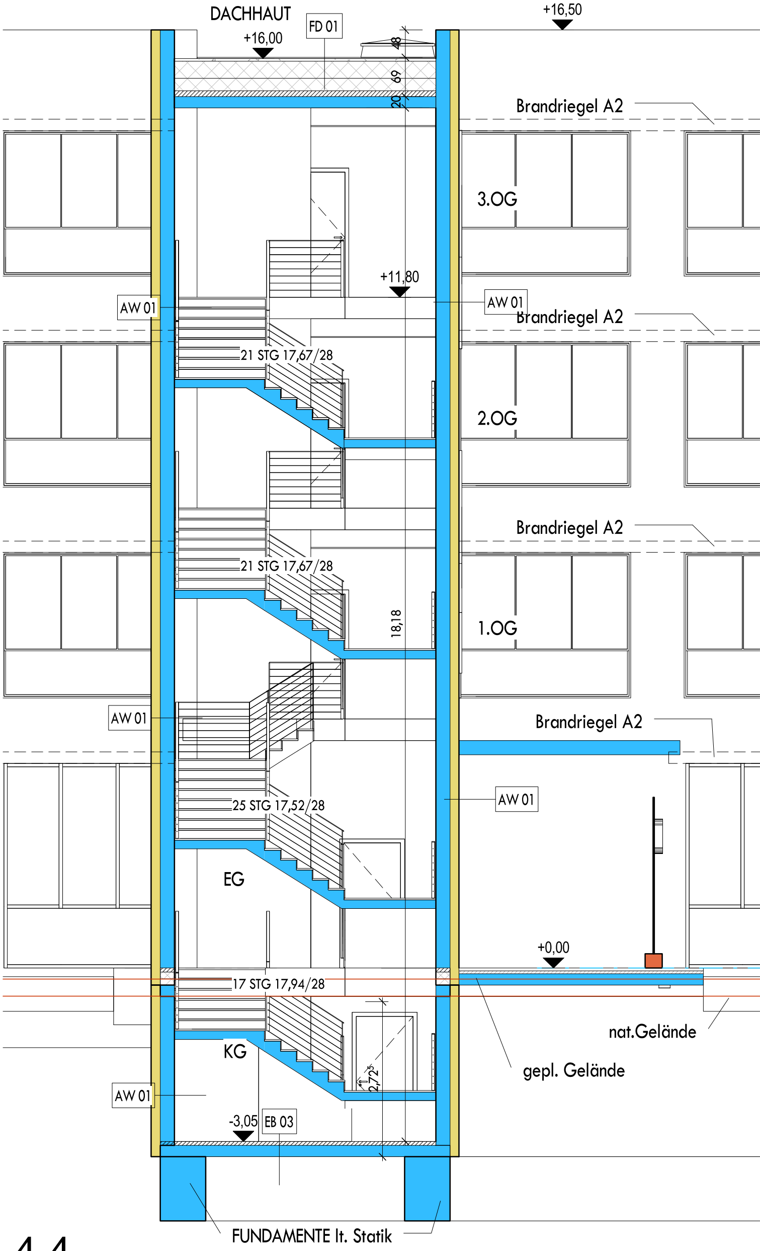
4-4 M 1 : 100
